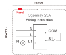
Fig. 1.110-240 V~ Power supply Abb. 1. 110-240 V~ Stromversorgung Fig. 1. Alimentazione 110-240 V~
